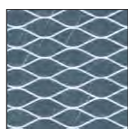
Wire : 1.8mm SWD: 12mm LWD: 23mm
